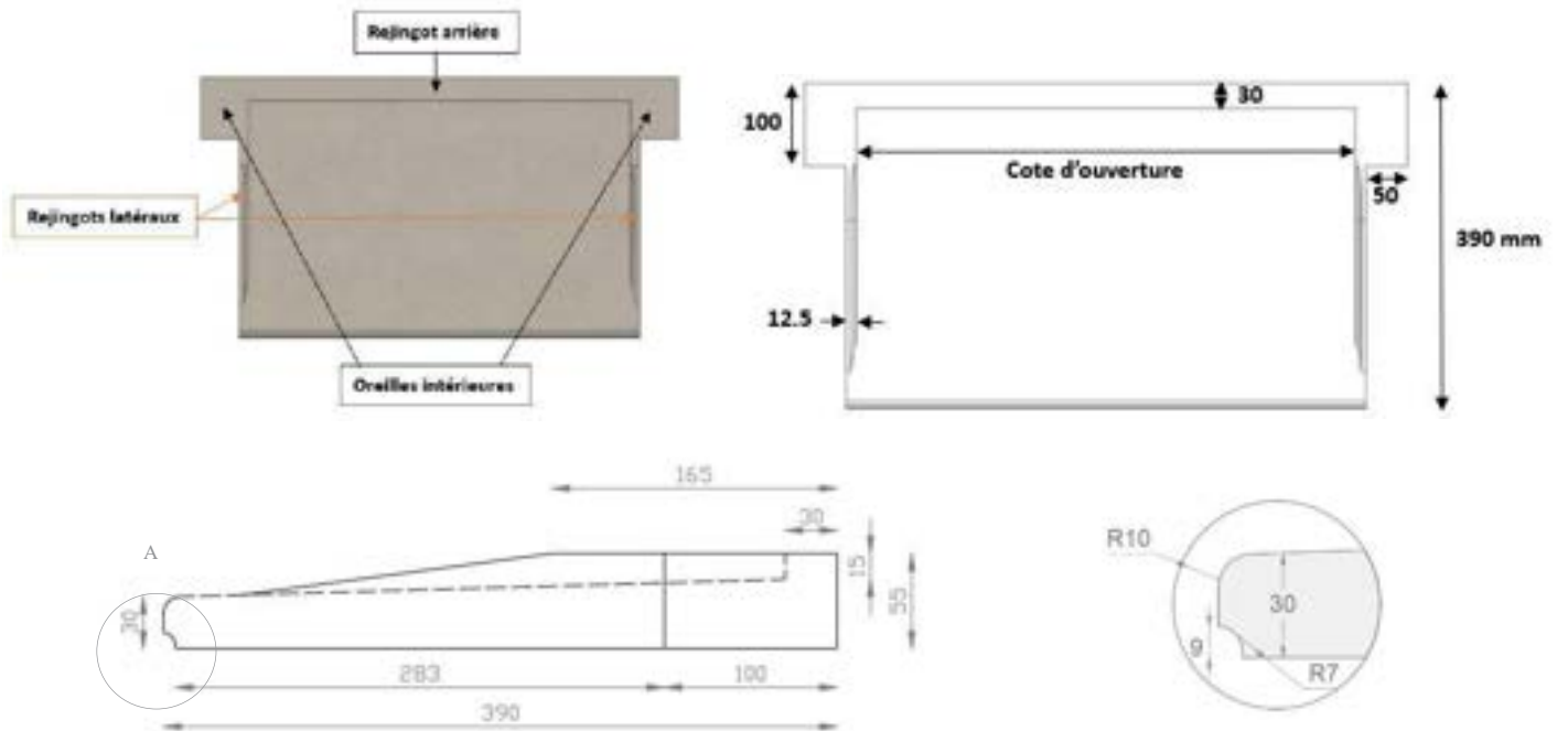
Vue en détail A
